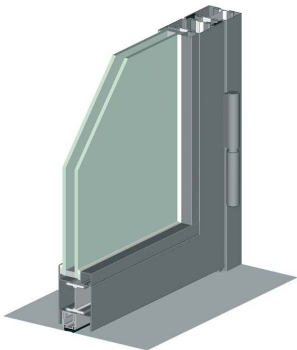
Sezione con profilo a taglio termico
